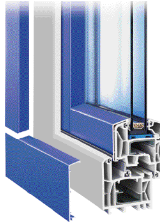
Modell hilzinger Innotherm-Alucolor, System Mitteldichtung, 70mm Bautiefe, flächenversetzt mit lichtgrauen Dichtungen und äußerer Aluminiumschale.
